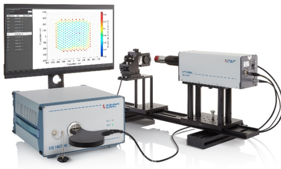
Abbildung: Die VTC 4000 ohne Faserausgang ermöglicht die Bestimmung von Leistung, Polarisation und Abstrahlcharakteristik der Einzelemitter. Mit zusätzlichem Faserausgang ist auch die Analyse der Wellenlängen mit Spektrometer möglich.
